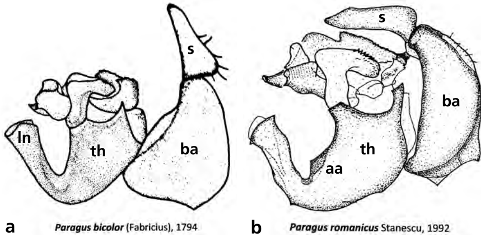
Fig. 1. Vues latérales des terminalia mâles de deux espèces de Paragus très proches: a ) P. bicolor (d'après Goeldlin 1976) et b ) P. romanicus (d'après Stănescu 1992). Abréviations: aa =processus de l'aedeage, s =surstylus du basale de l'hypopygium, ba =épandrium (basale), ln =lingula de la thèque de l'hypopygium, th =thèque de l'hypopygium.
